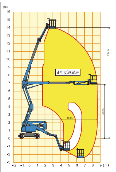
■NUL14WJ作業範囲図
