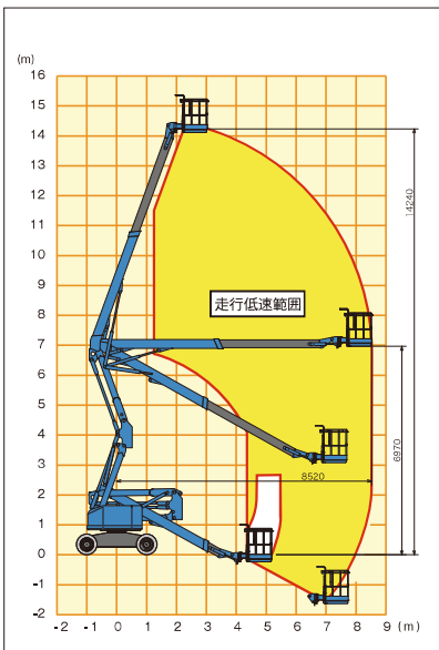
■NUL14W作業範囲図
