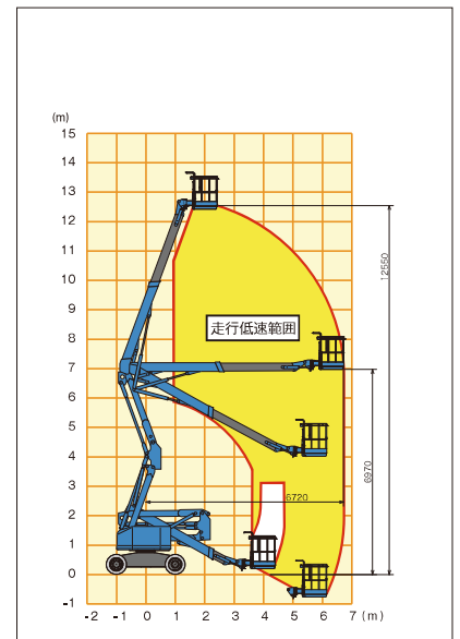
■NUL12W作業範囲図
