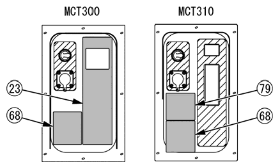
P部詳細 (ラジコン受信部)
