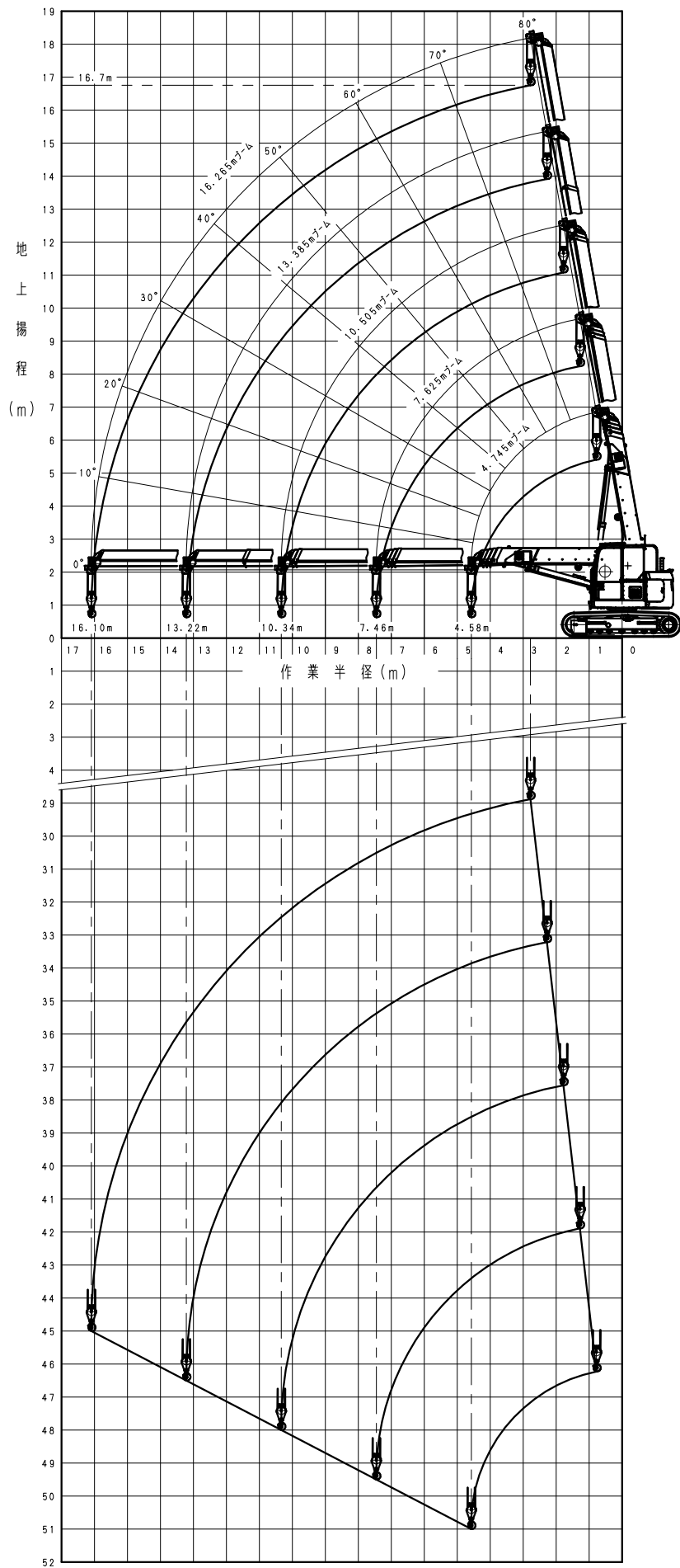
CC1485S-1 作業半径揚程図(2本掛け)
