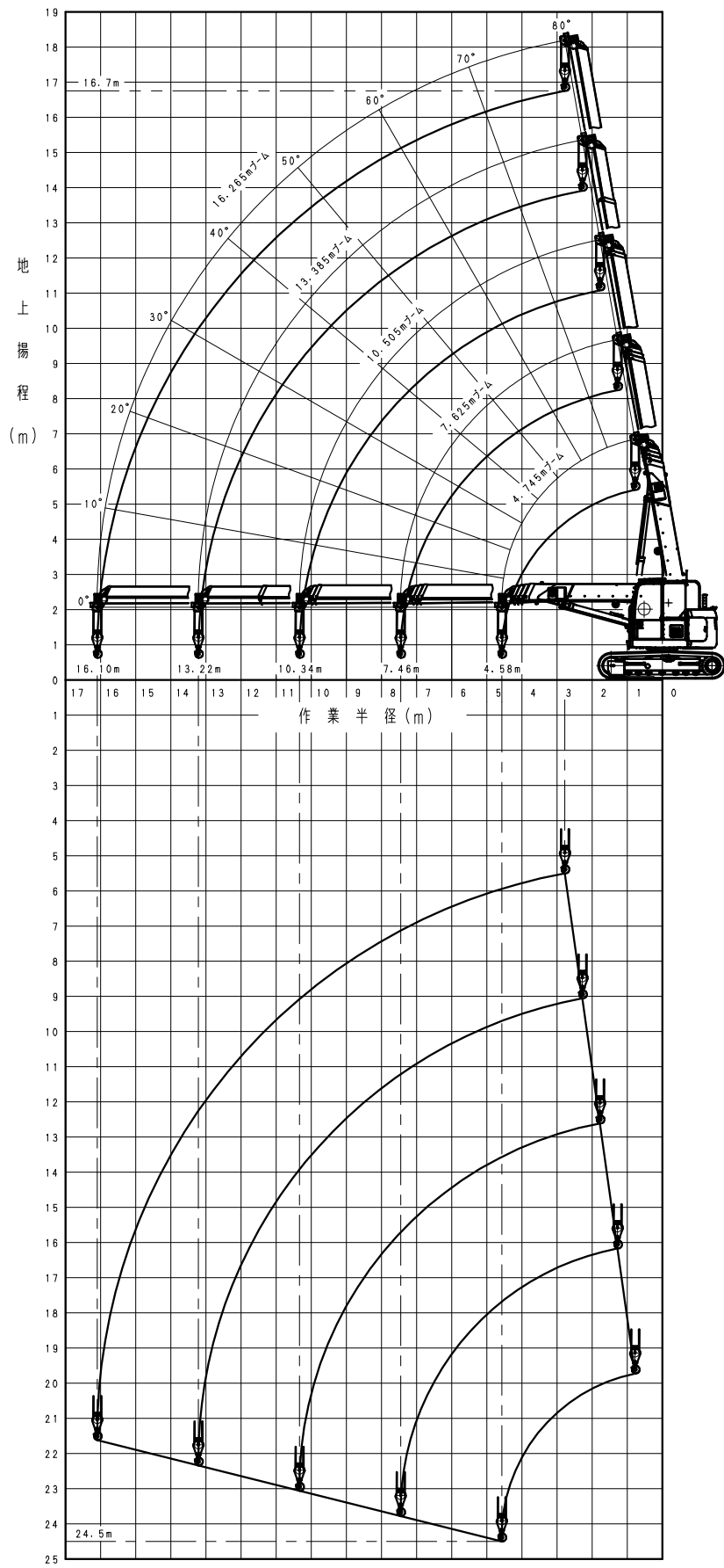
CC1485S-1 作業半径揚程図 (4本掛け)
